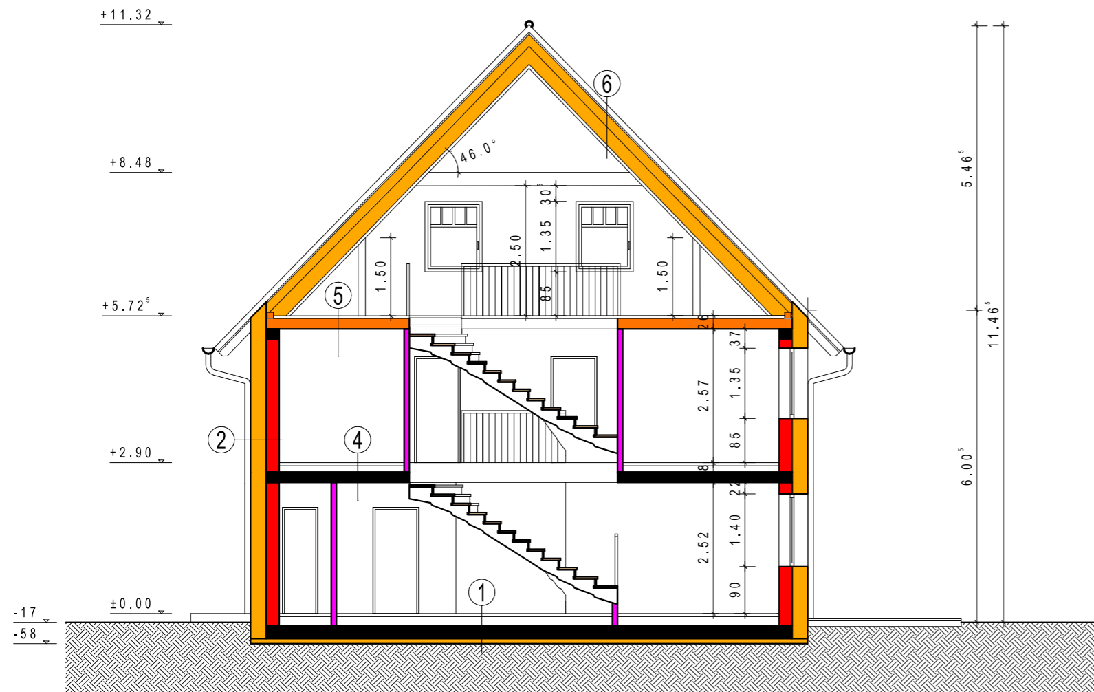
SCHNITT A-A
